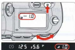
Indicateur d'état d'exposition
