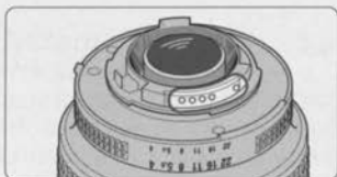
Contacts UCT d'un objectif à microprocesseur
